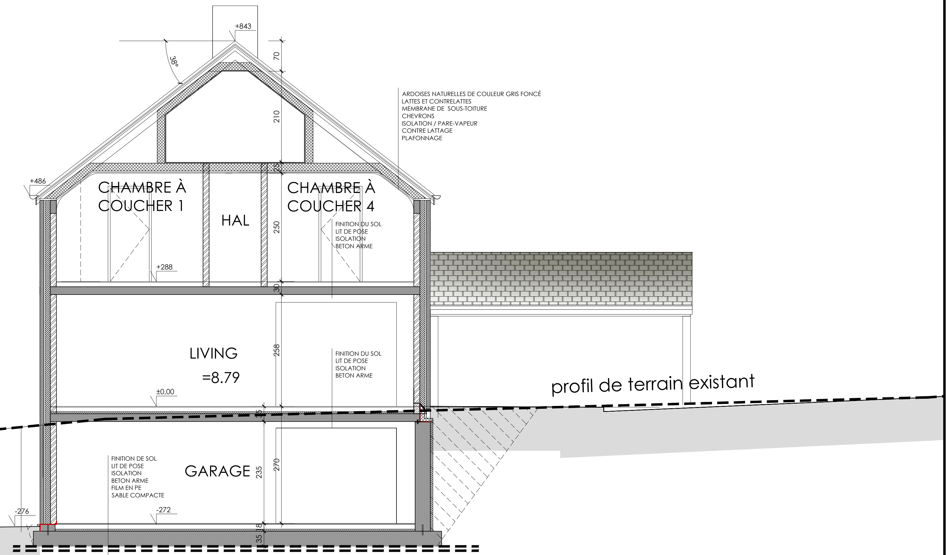
COUPE A-A
