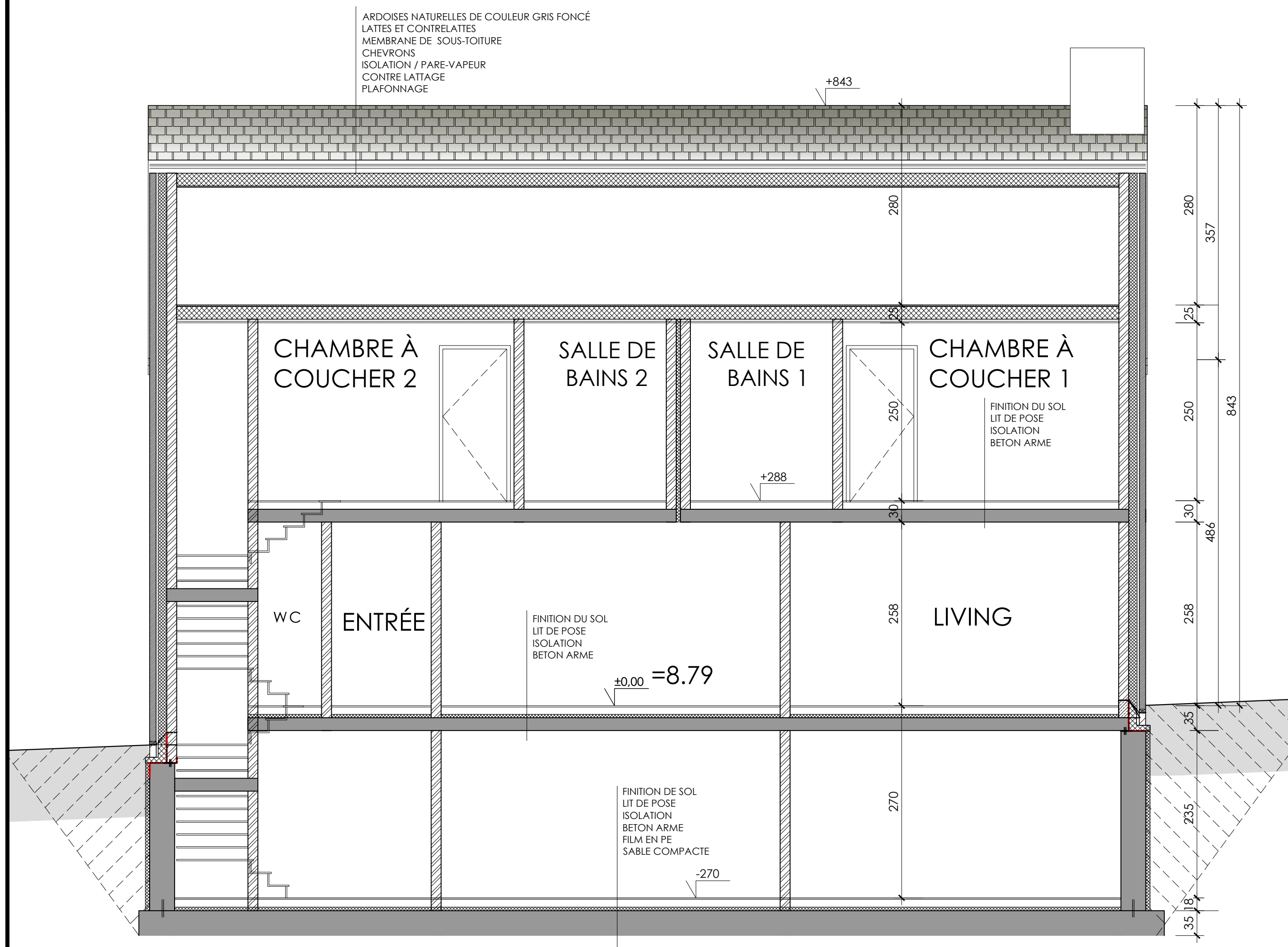
COUPE B-B
